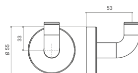
Hook matte black
